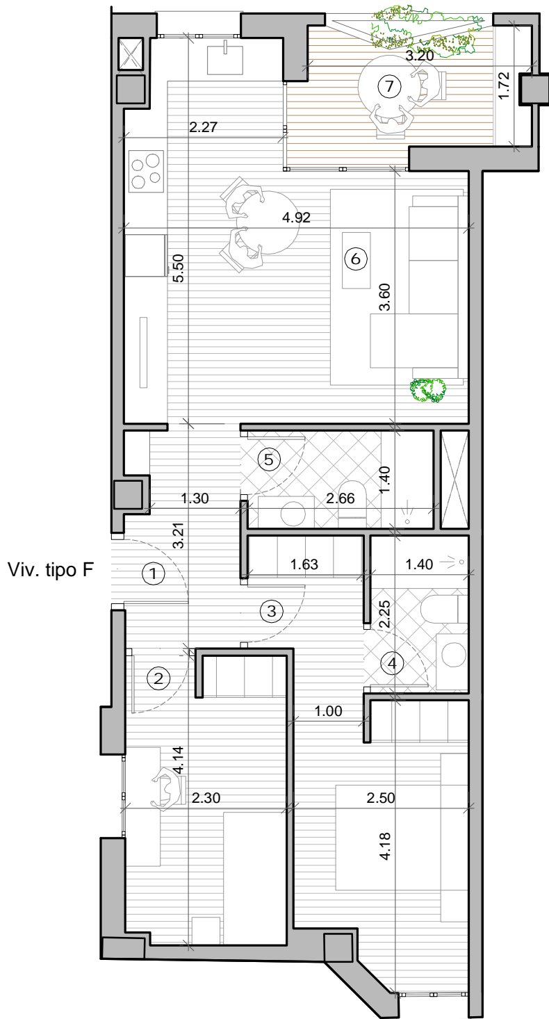
VIVIENDA TIPO F Escala 1:75
